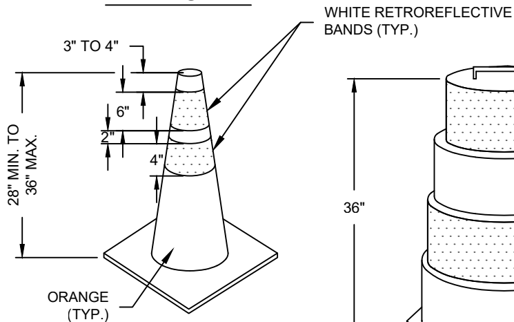
CONE
