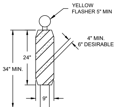
CONE
