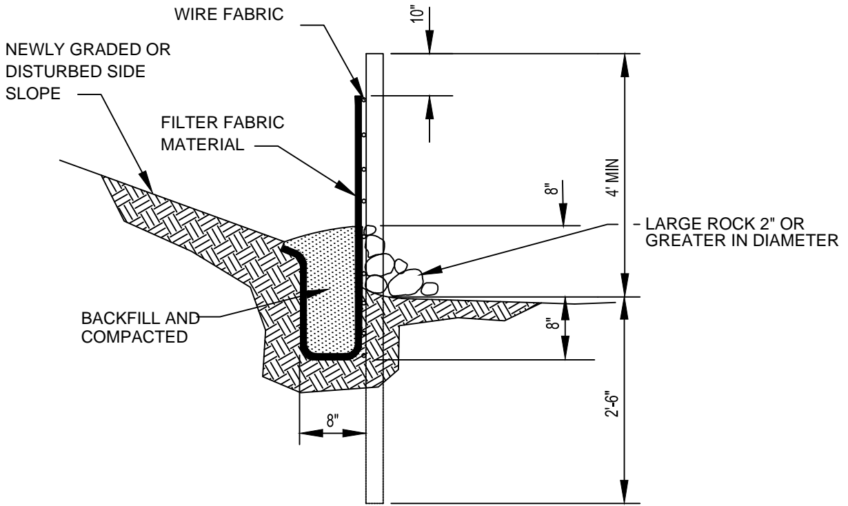
SECTION A-A
